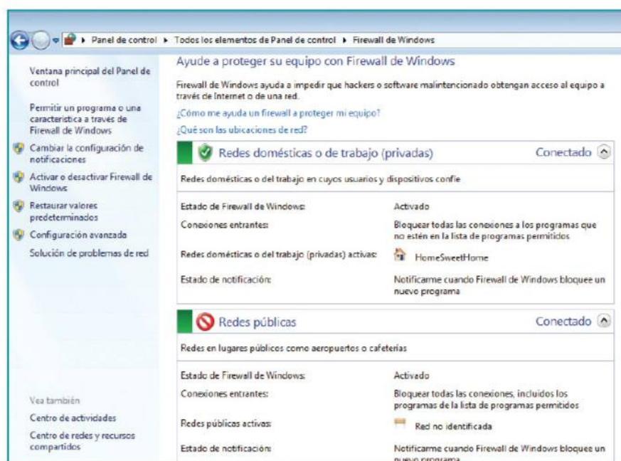
En esta imagen podemos ver el panel de administración del Firewall de Windows 7; en él se indica el perfil activo.
