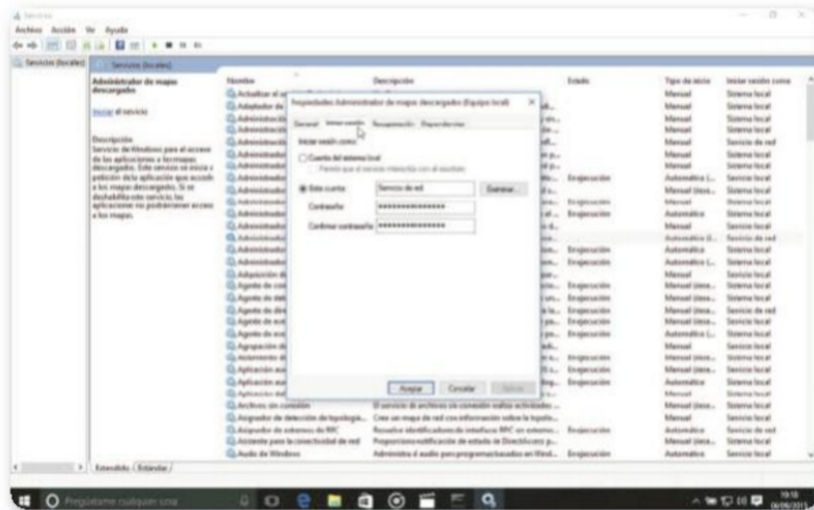
Figura 10. En la pestaña Iniciar sesión podemos especificar bajo qué permisos de usuario se ejecutará un servicio y el perfil de hardware adecuado.
