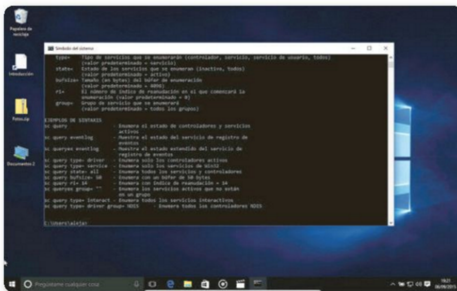
Figura 12. Si escribimos SC en el intérprete de comandos, tendremos acceso a un listado completo de las funciones que esta aplicación nos entrega.
