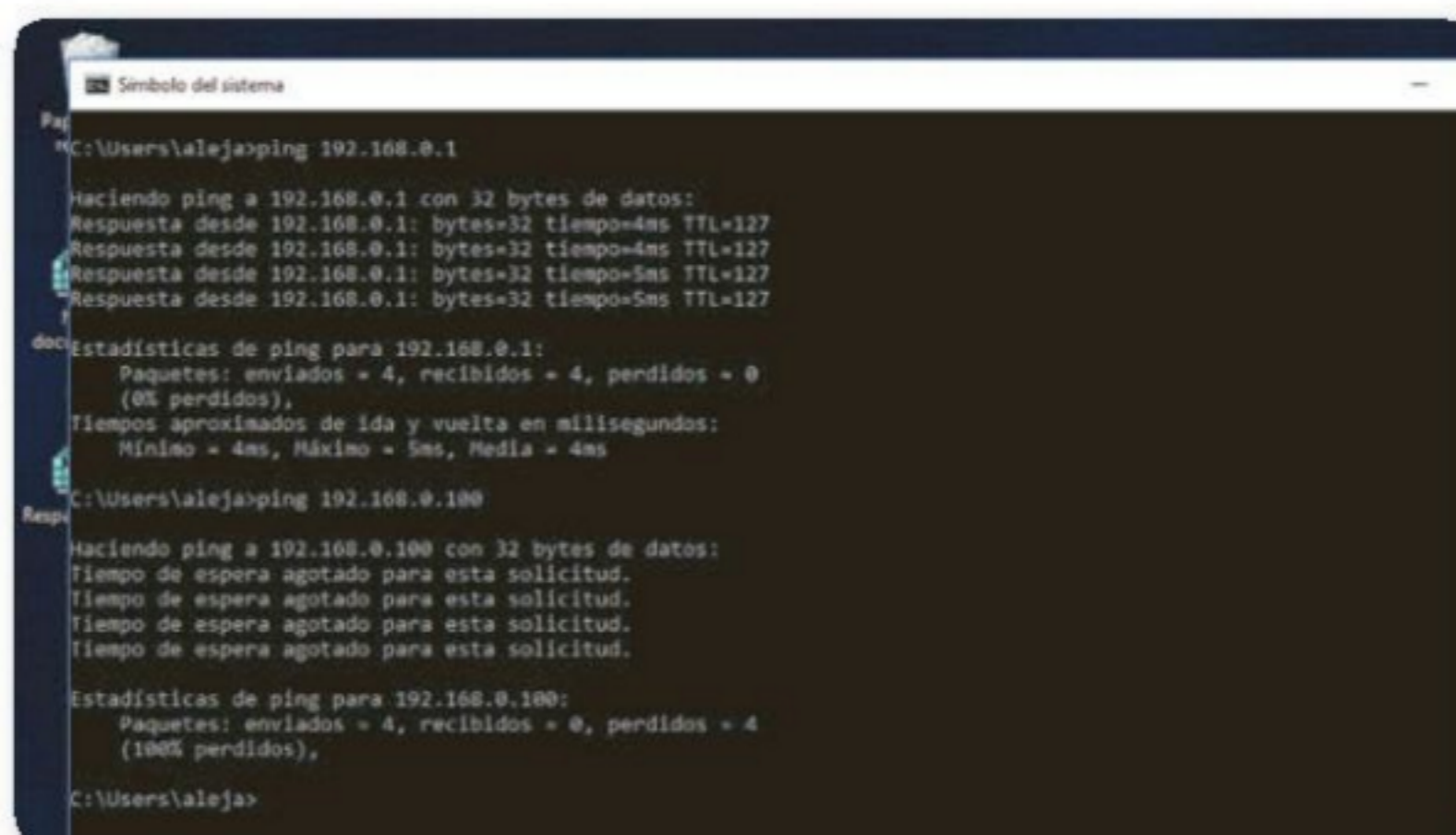
Figura 18. Para probar la comunicación con otro equipo ejecutamos el comando PING con la dirección IP adecuada. Un error indica que el equipo no se encuentra disponible o que no estamos conectados.
