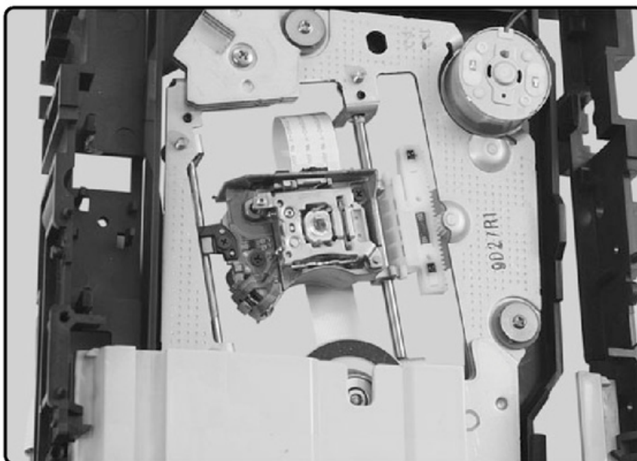
FIGURA 3. La bandeja de las unidades ópticas suelen tener bastantes inconvenientes luego de una prolongada utilización o incluso el hecho de no utilizarse hará que la correa de transmisión del mecanismo se estire.
