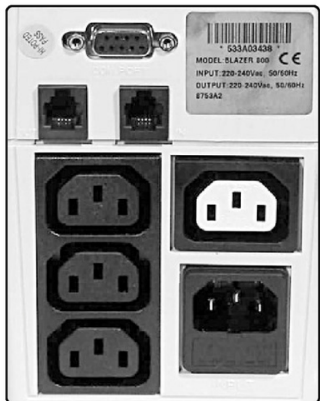
FIGURA 5. En esta imagen, observamos la parte trasera de una unidad UPS o SAI. Algunos modelos incluyen salidas de 110 y 220 voltios.
