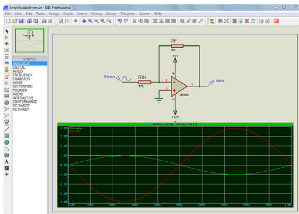
► Figura 2. El gráfico mostrará las señales analógicas generadas en los puntos elegidos en el circuito.
