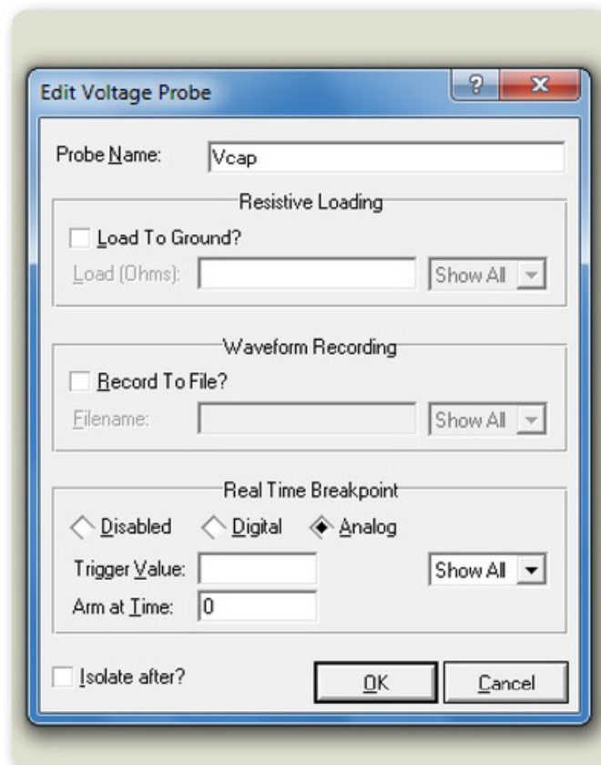
▶ Figura 15. Las sondas de voltaje pueden servir como puntos de ruptura analógicos o digitales.
