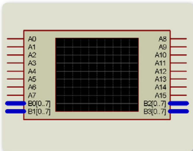
Figura 11. El analizador lógico cuenta con 16 canales individuales (A0 a A15) y 4 analizadores de buses (B0 a B3).
