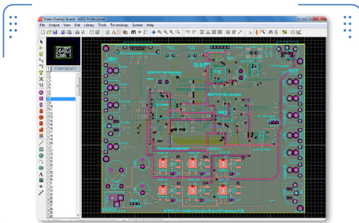
► Figura 3. El módulo ARES permite el diseño de circuitos impresos donde construiremos los circuitos de forma física.
