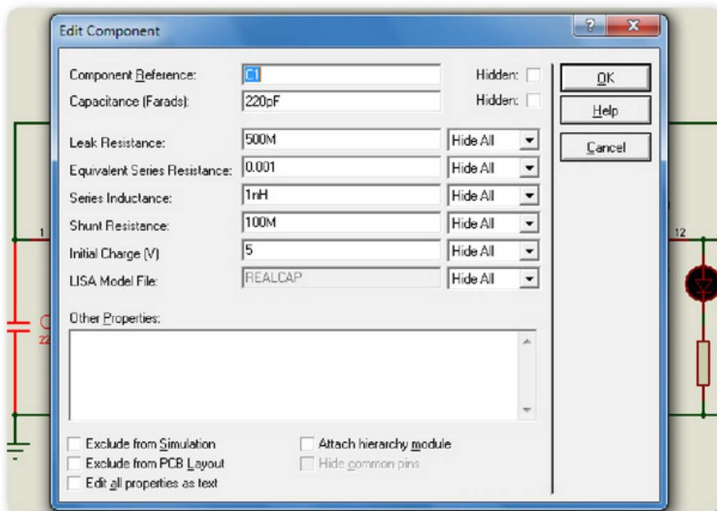
► Figura 21. El modelo REALCAP es un capacitor que se asemeja mucho al comportamiento de un capacitor verdadero.
