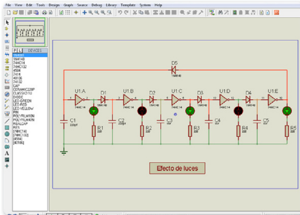
► Figura 20. Un efecto de luces con LEDs es un interesante ejemplo de un circuito mixto de tipo sencillo.
