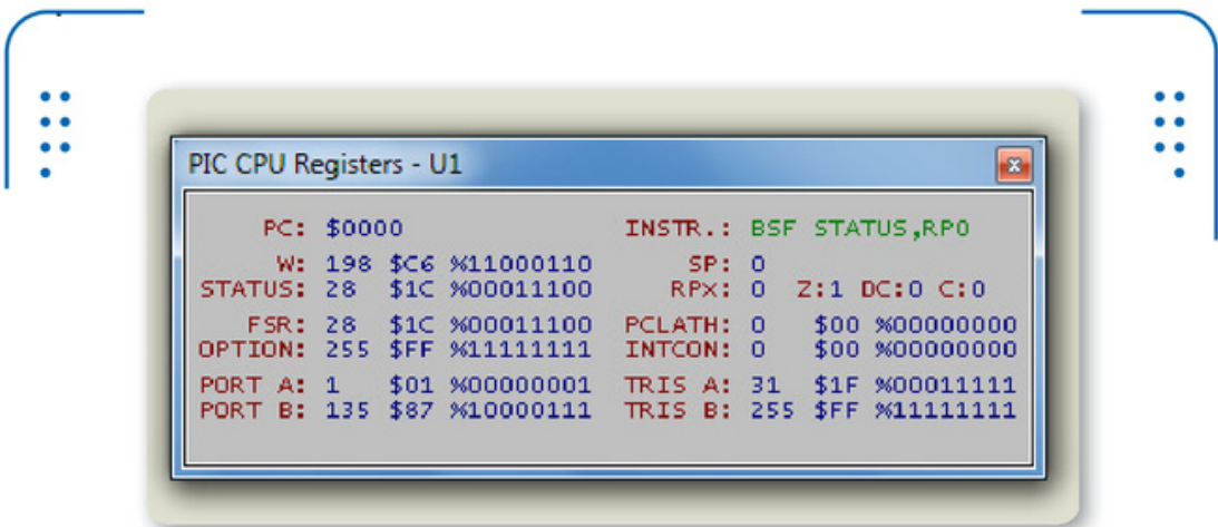
Figura 10. El contenido de la ventana PIC CPU Registers en el ejemplo del contador binario.
