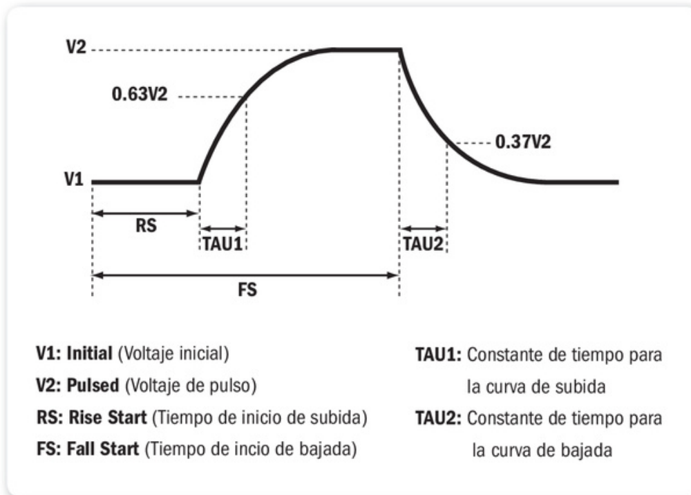
► Figura 9. Podemos construir una señal exponencial definiendo sus parámetros con el generador EXP.
