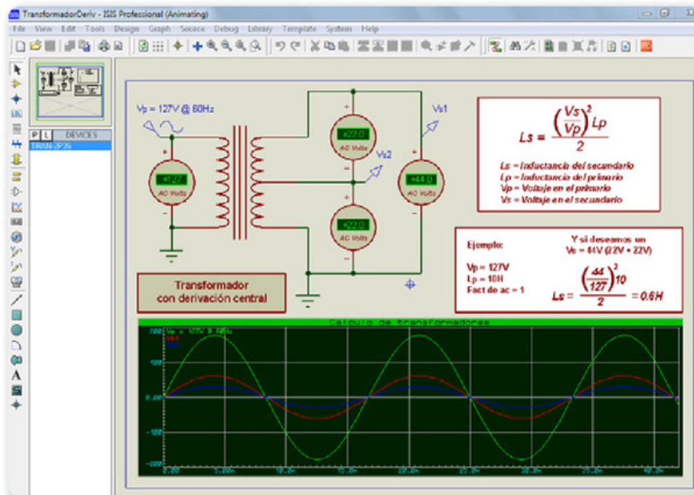
► Figura 7. Los transformadores con derivación central también pueden ser calculados para un valor específico a la salida.
