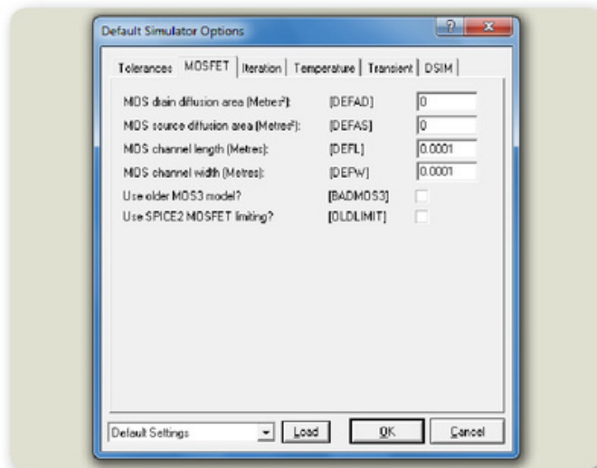
► Figura 6. La pestaña MOSFET nos permite establecer parámetros para este tipo de transistores.
