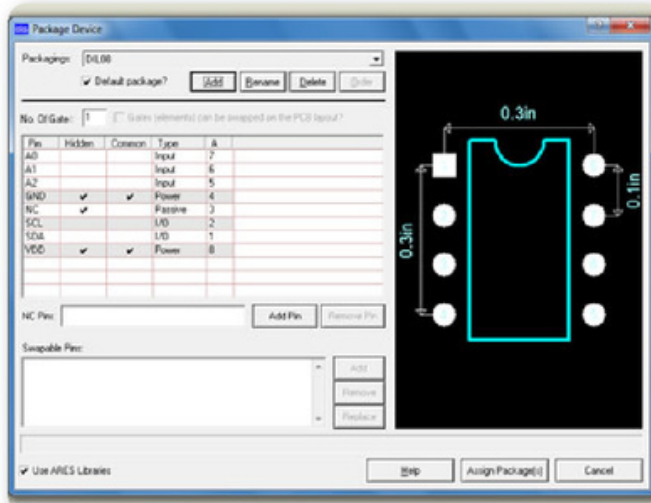
► Figura 17. El empaque DIL08 ya asignado en la herramienta visual de empaques.
