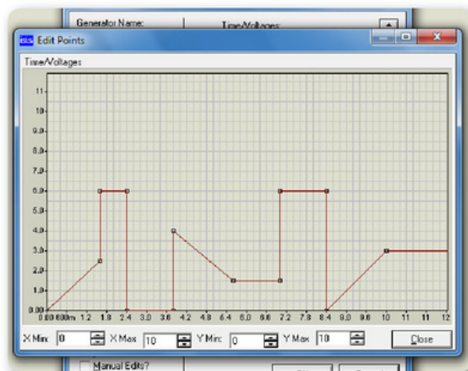
Figura 10. Ejemplo del gráfico del generador PWLIN expandido y con una señal dibujada en él.
