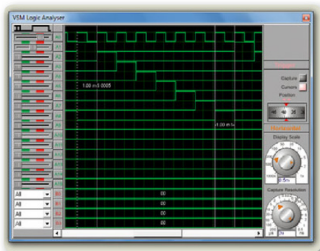
► Figura 13. Podemos ver el funcionamiento del circuito integrado 4022 usando el analizador lógico.
